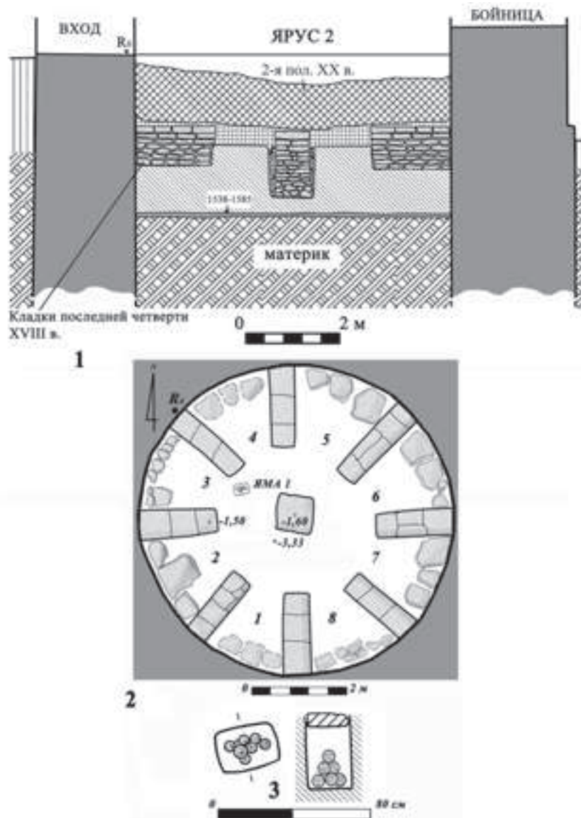
Рис. 2. 1 – разрез нижнего яруса башни по линии северо-запад – юго-восток; 2 – план нижнего яруса; 3 – яма 1
